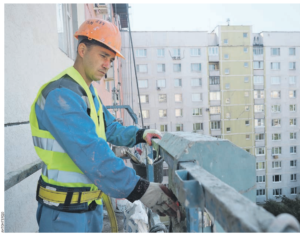
29 августа 2019 года 15:17 Мастер Виктор Никишин в специальной строительной люльке проводит ремонт фасада по современной технологии
