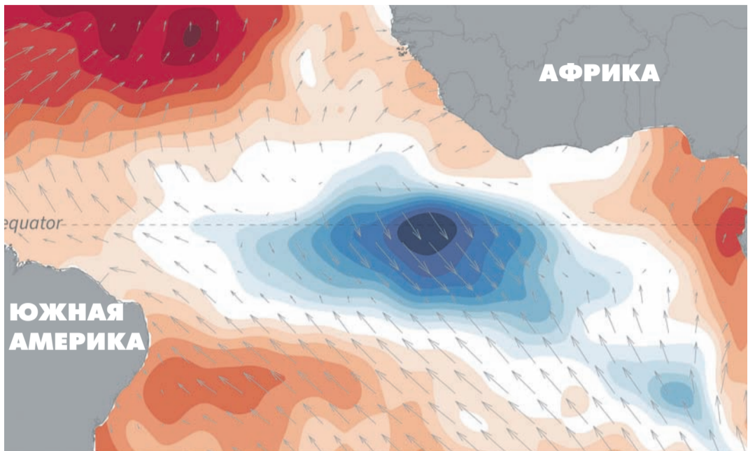
Температурная аномалия в Атлантическом океане
