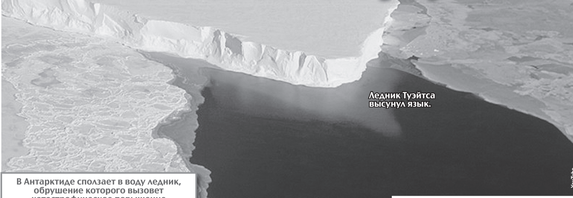
ЛЕДНИК ТУЭЙТСА
